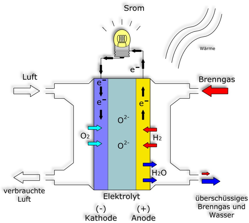
Abb.01: Prinzip-Skizze einer Brennstoffzelle (Copyright: Dieter Rieger)
